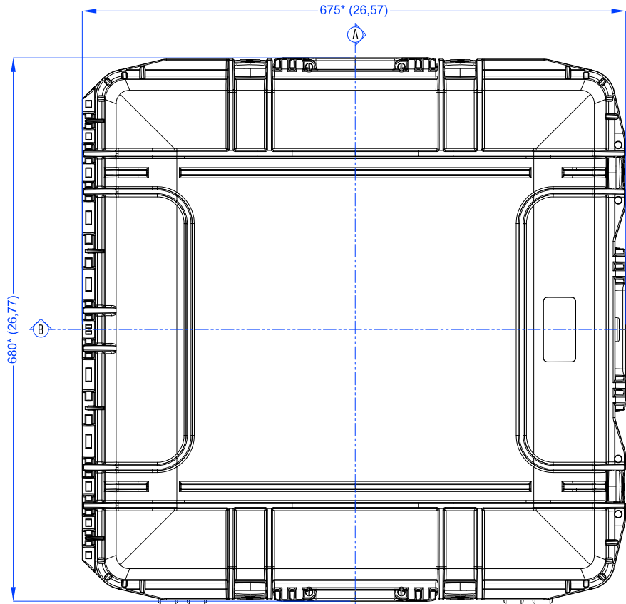
Vista Coperchio
