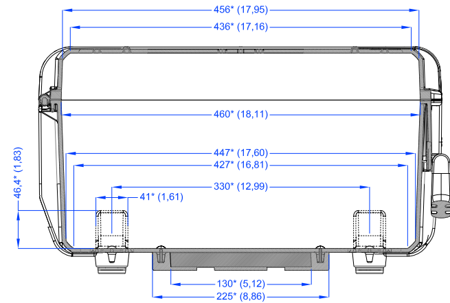
Sezione B-B Section B-B
