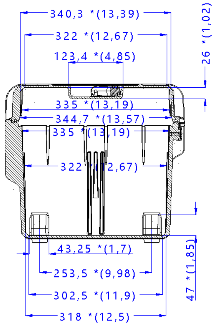
Sezione B-B Section B-B
